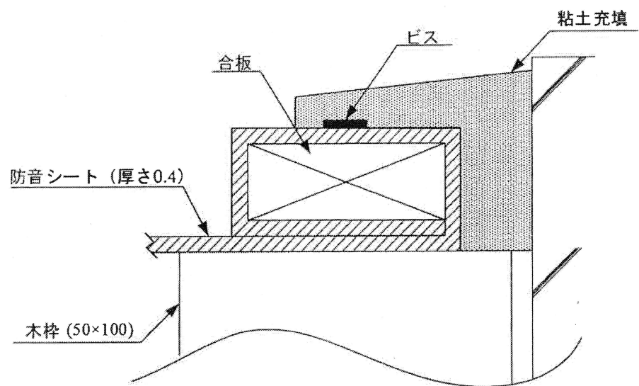
端部詳細断面図
