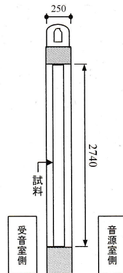
試験開口断面
