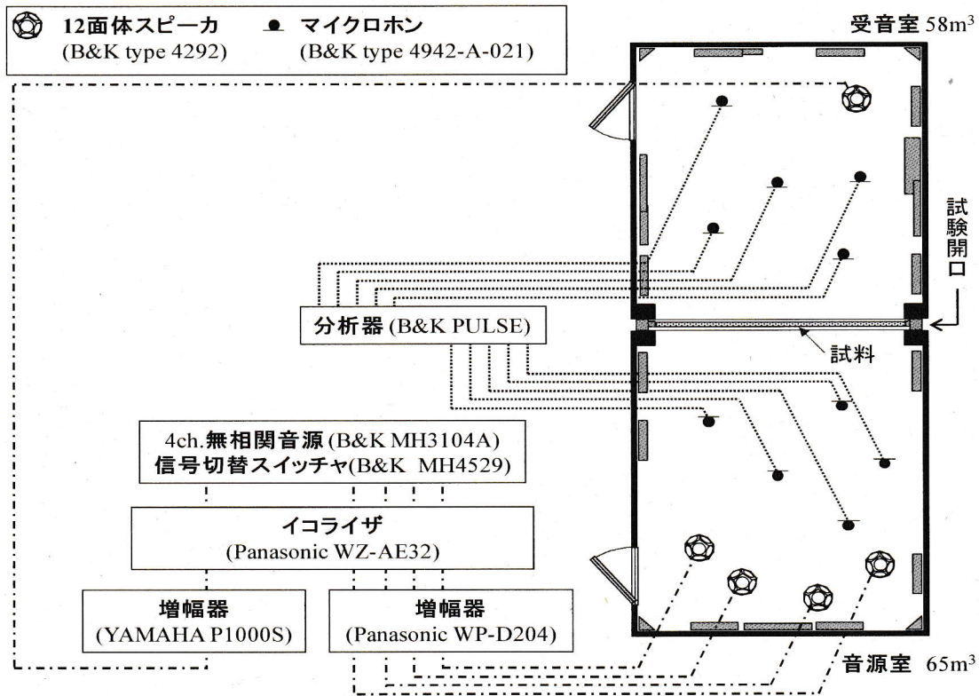
タイプII試験室および測定装置
